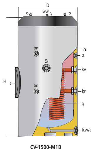
CV-1500-M1B
