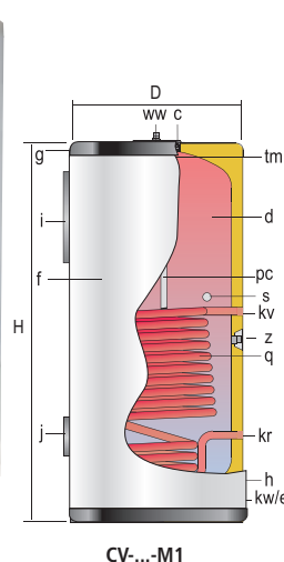
CV-...-M1
